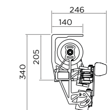
Jade bras croisés Pose Plafond
