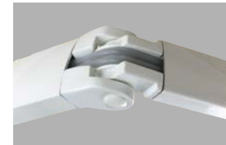
Bras testés à 20 000 cycles dotés d'une articulation à double câble gainé.
