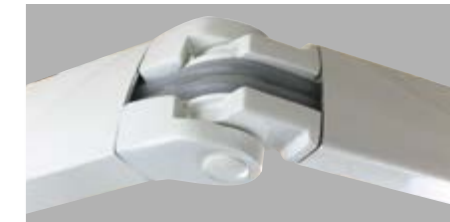
Bras testés à 20 000 cycles dotés d'une articulation à double câble gainé.
