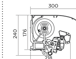
Perle et Perle Lux Pose Face avec auvent
