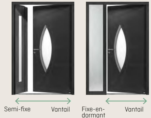
← Largeur de passage → Prado Duo : double vantaux, imposte à motif coordonné et semi-fixe. Prado Duo : porte avec imposte pleine en faux ouvrant.
