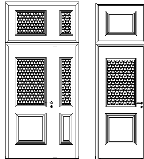
← Largeur de passage → Prado Duo : double vantaux, imposte à motif coordonné et semi-fixe. Prado Duo : porte avec imposte pleine en faux ouvrant.
