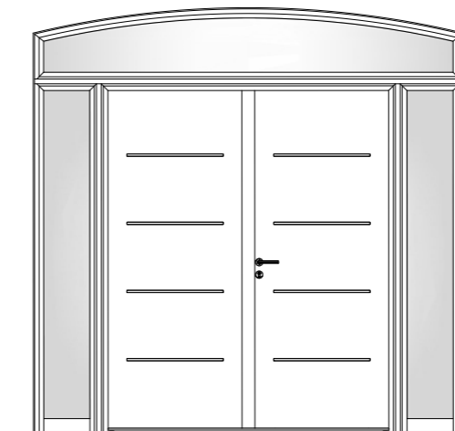
← Largeur de passage → Cotim 11 Duo : double vantaux, 2 fixes en dormant vitrés et imposte vitrée arc surbaissé.
